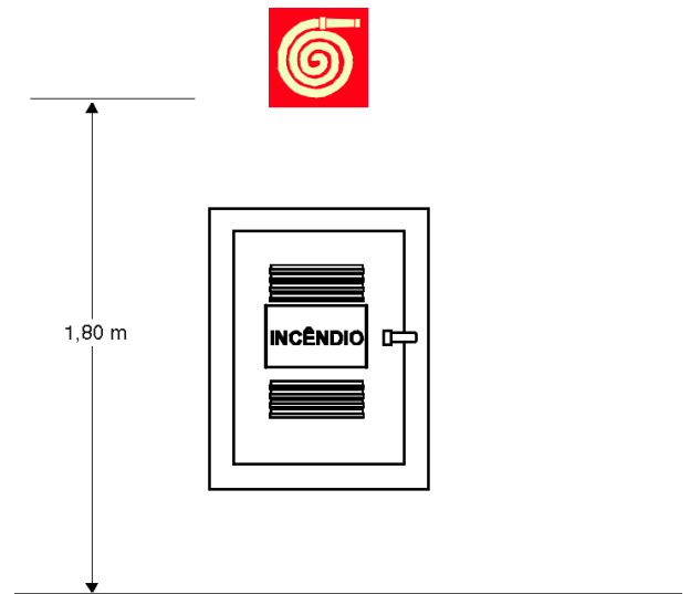
Figura 7 - Sinalização de hidrante
